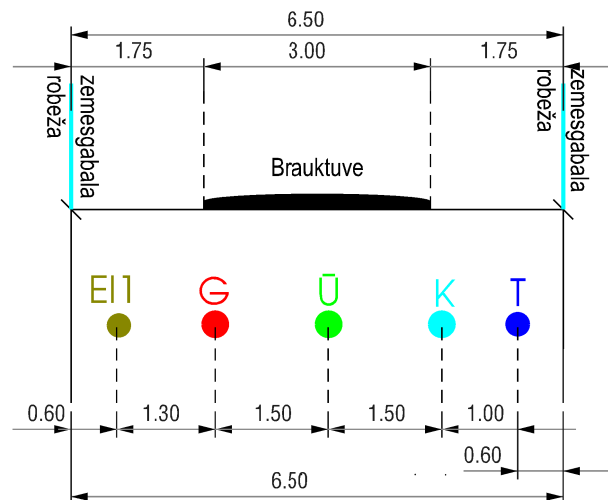
PIEBRAUCAMĀ CEĻA PROFILS B-B
