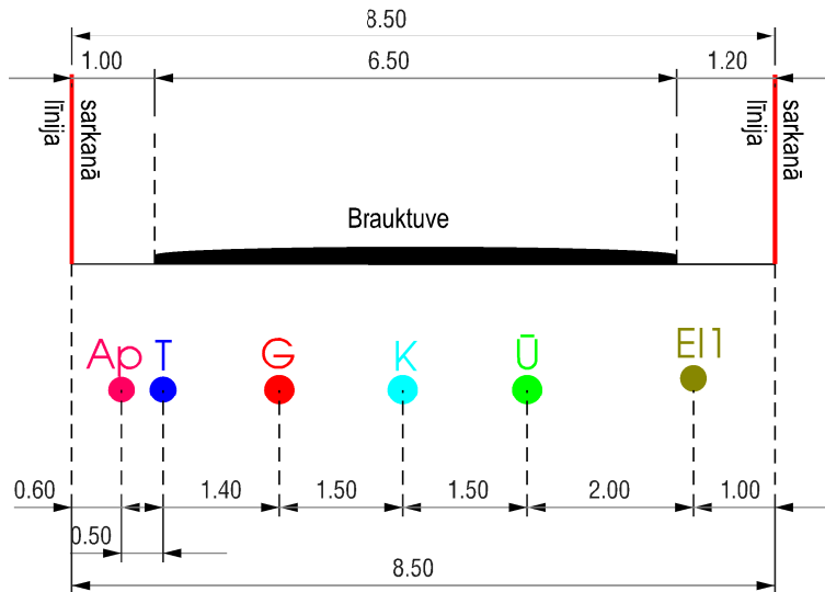
SALACAS IELAS PROFILS A-A
