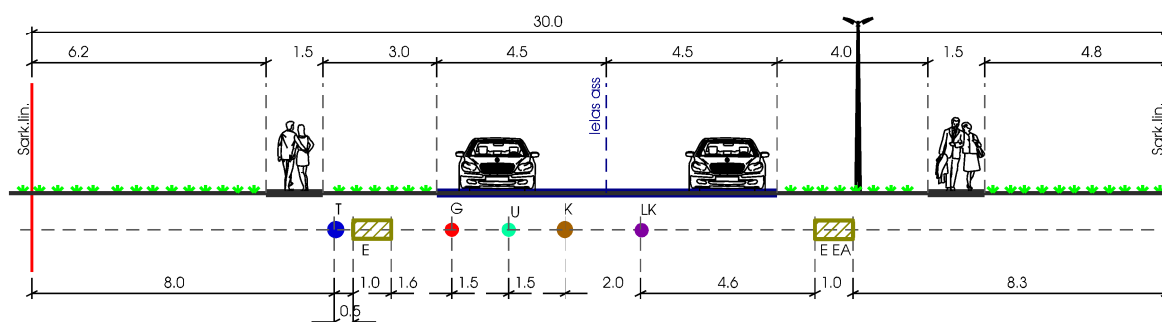
griezums A - A Rīgas ielas sarkanās līnijas 30.0m
