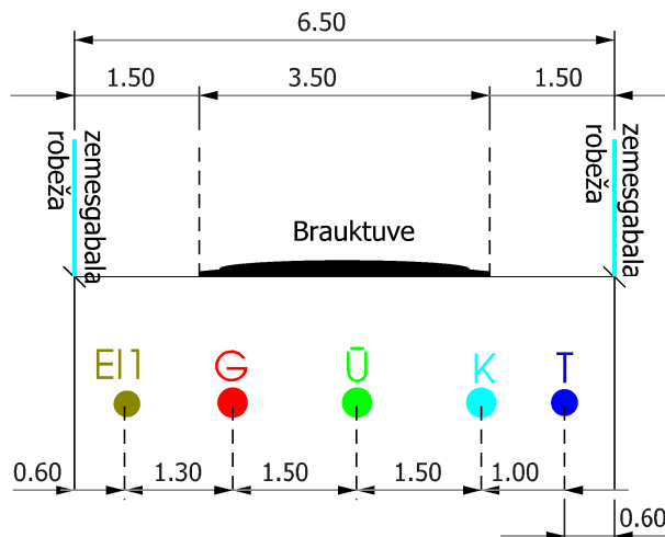
PIEBRAUCAMĀ CEĻA PROFILS (plānotais) GRIEZUMS B-B
