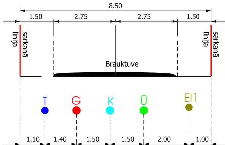
SALACAS IELAS PROFILS GRIEZUMS A-A
