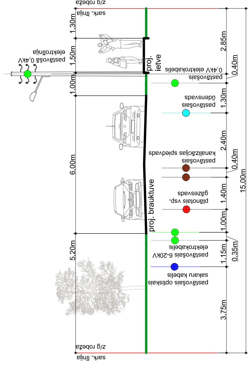
Apes iela, sarkanās līnijas 15,0m, D2 kategorijas iela, griezums A-A
