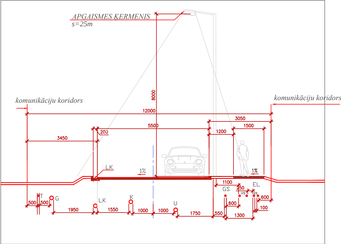
PROJEKTĒJAMĀ PIEBRAUCAMĀ CEĻA ŠĶĒRSPROFILS 2-2
