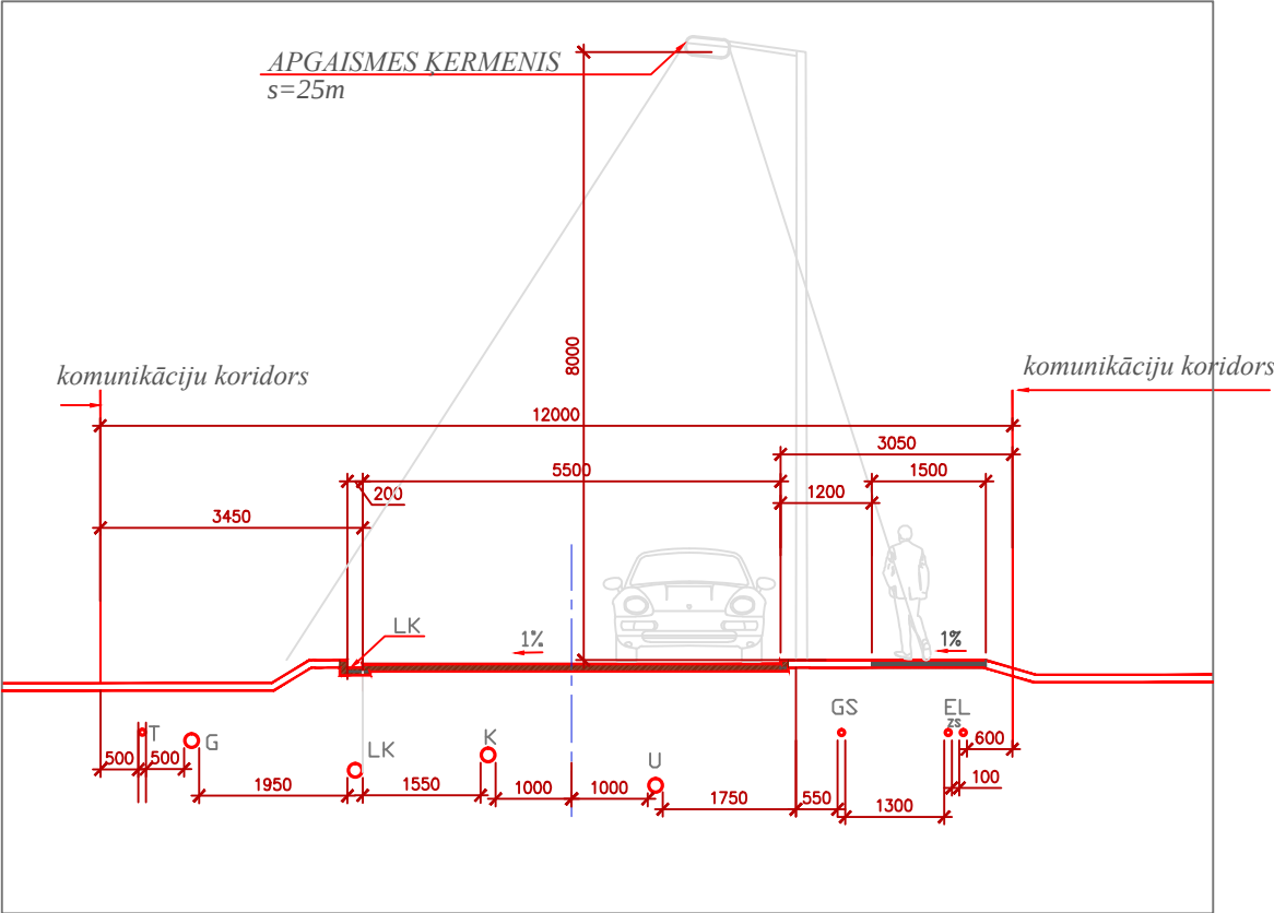
PROJEKTĒJAMĀ PIEBRAUCAMĀ CEĻA ŠĶĒRSPROFILS 1-1
