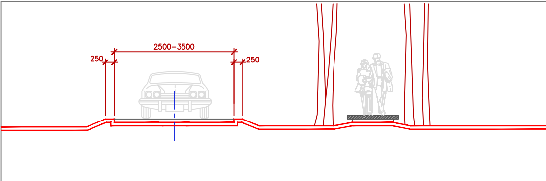
PROJEKTĒJAMĀ PIEBRAUCAMĀ CEĻA ŠĶĒRSPROFILS 3-3*
