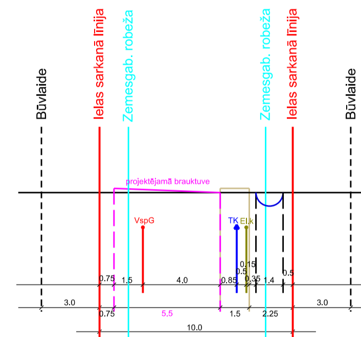
Dzērveņu ielas šķērsprofils 17-17 M 1:285
