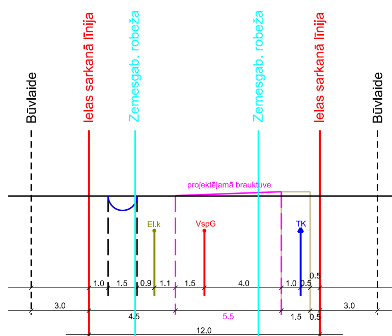
Bažciema ielas šķērsprofils 20-20 M 1:285
