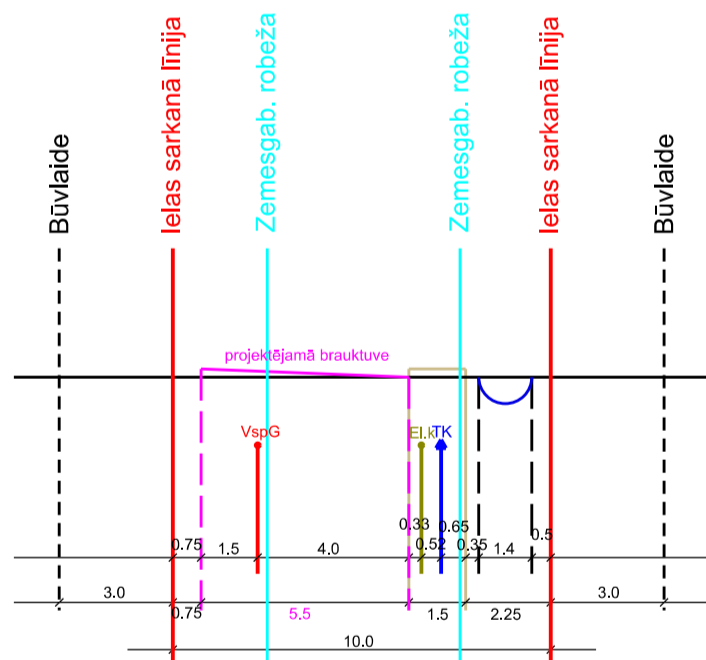
Rapšu ielas šķērsprofils 13-13 M 1:285
