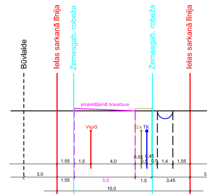
Dzērveņu ielas šķērsprofils 16-16 M 1:285
