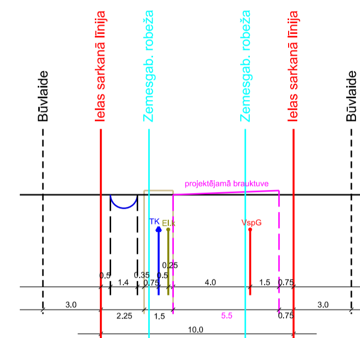
Dadžu ielas šķērsprofils 10-10 M 1:285
