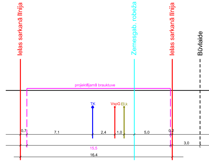
Bārbeļu ielas šķērsprofils 1-1 M 1:285
