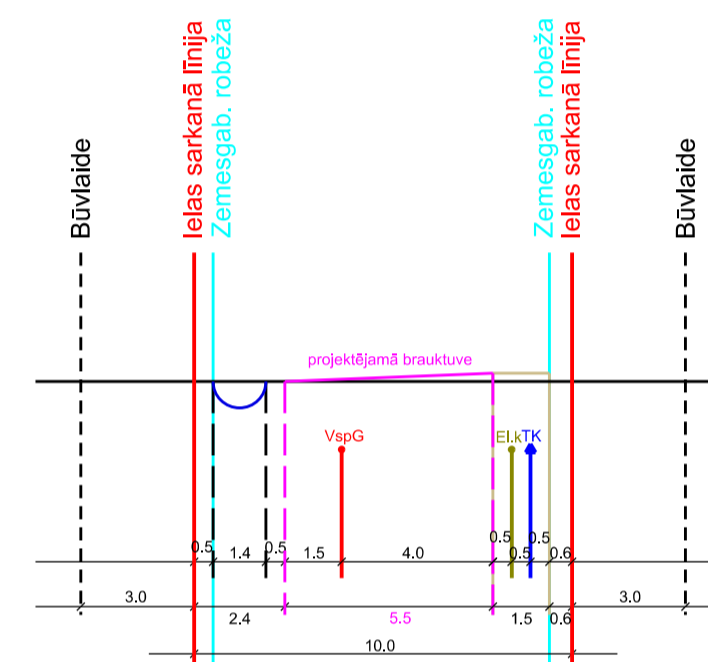
Dadžu ielas šķērsprofils 12-12 M 1:285
