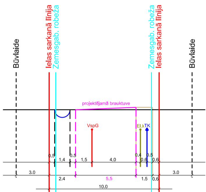
Rapšu ielas šķērsprofils 14-14 M 1:285
