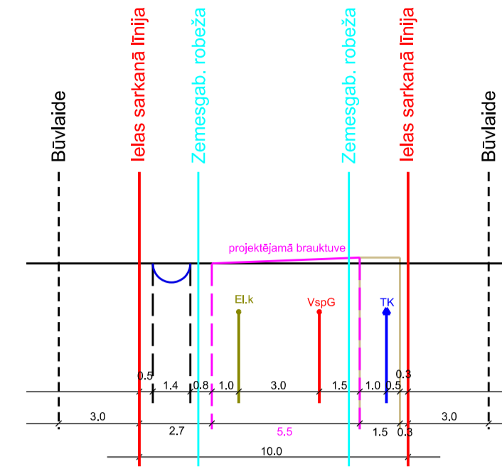
Circeņu ielas šķērsprofils 5-5 M 1:285
