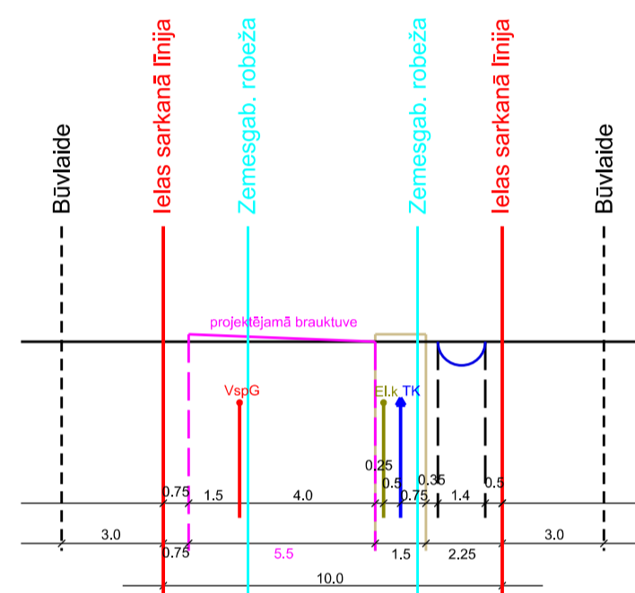
Dadžu ielas šķērsprofils 9-9 M 1:285
