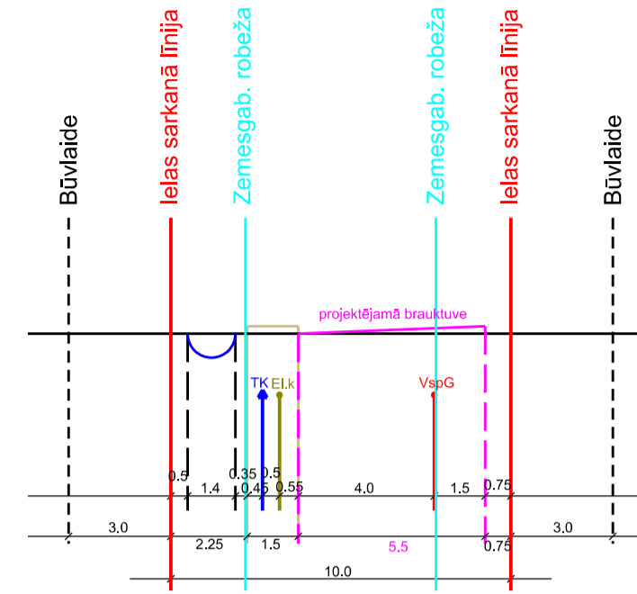
Circeņu ielas šķērsprofils 6-6 M 1:285
