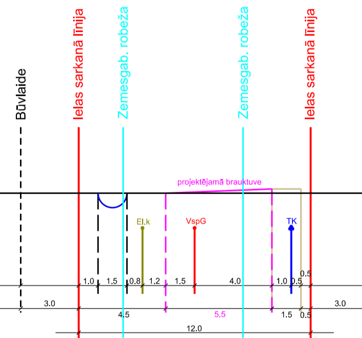
Bažciema ielas šķērsprofils 18-18 M 1:285
