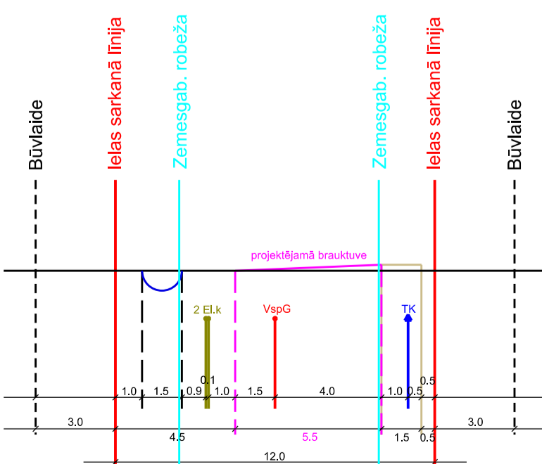
Bažciema ielas šķērsprofils 21-21 M 1:285
