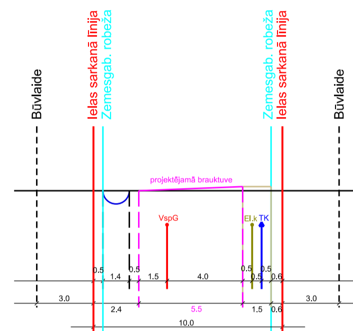
Dadžu ielas šķērsprofils 11-11 M 1:285
