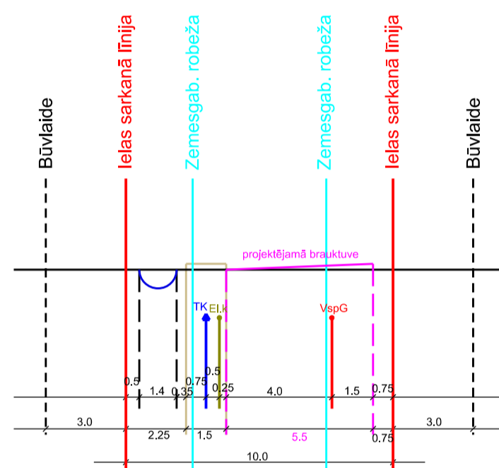
Dlomīta ielas šķērsprofils 7-7 M 1:285
