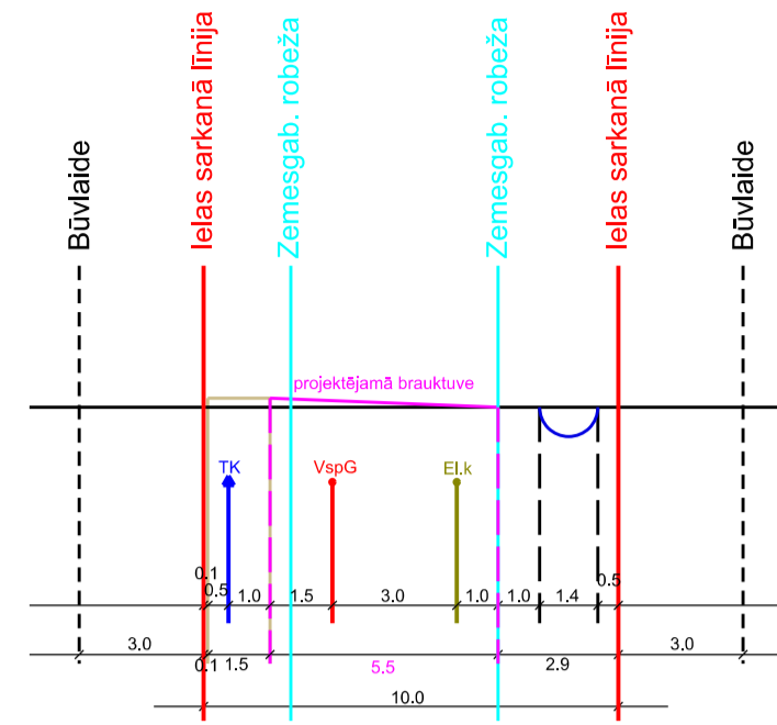
Circeņu ielas šķērsprofils 3-3 M 1:285
