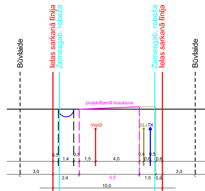
Rapšu ielas šķērsprofils 15-15 M 1:285
