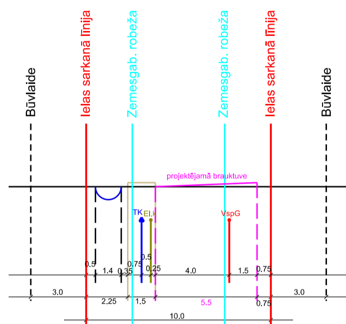
Dijļu ielas šķērsprofils 8-8 M 1:285
