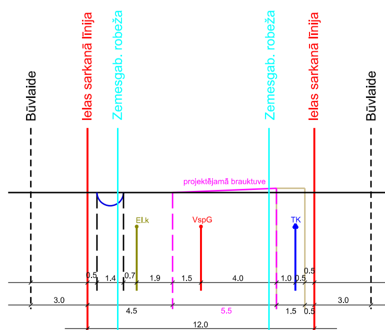
Bažciema ielas šķērsprofils 19-19 M 1:285
