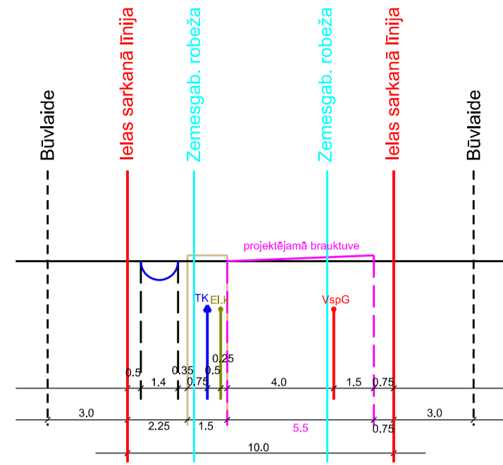
Bārbeļu ielas šķērsprofils 2-2 M 1:285
