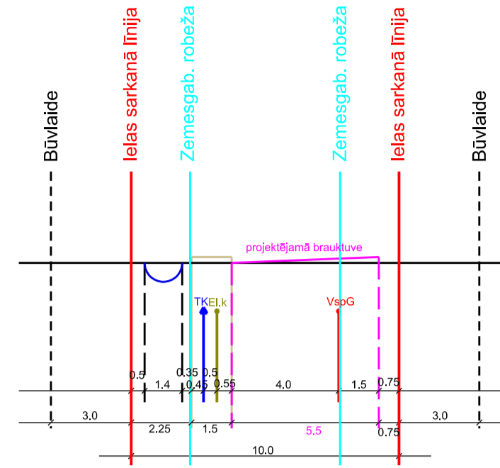
Circeņu ielas šķērsprofils 4-4 M 1:285
