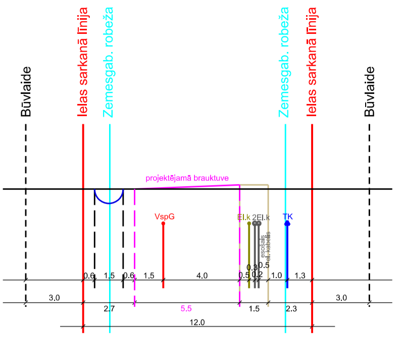
Līkloču ielas šķērsprofils 27-27 M 1:285
