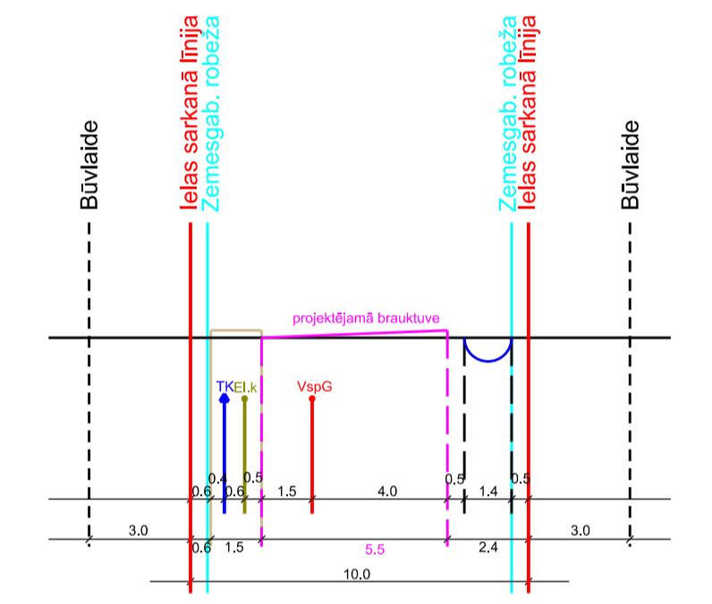
Līkloču ielas šķērsprofils 32-32 M 1:285
