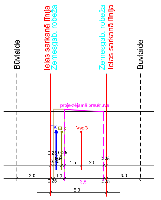
Piņņu ielas šķērsprofils 38-38 M 1:285
