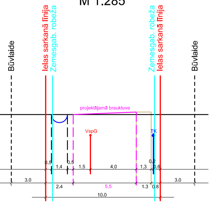
Seleriju ielas šķērsprofils 40-40 M 1:285
