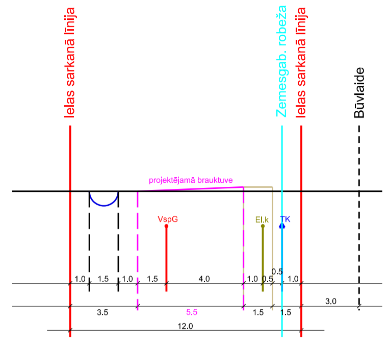
Bažciema ielas šķērsprofils 23-23 M 1:285
