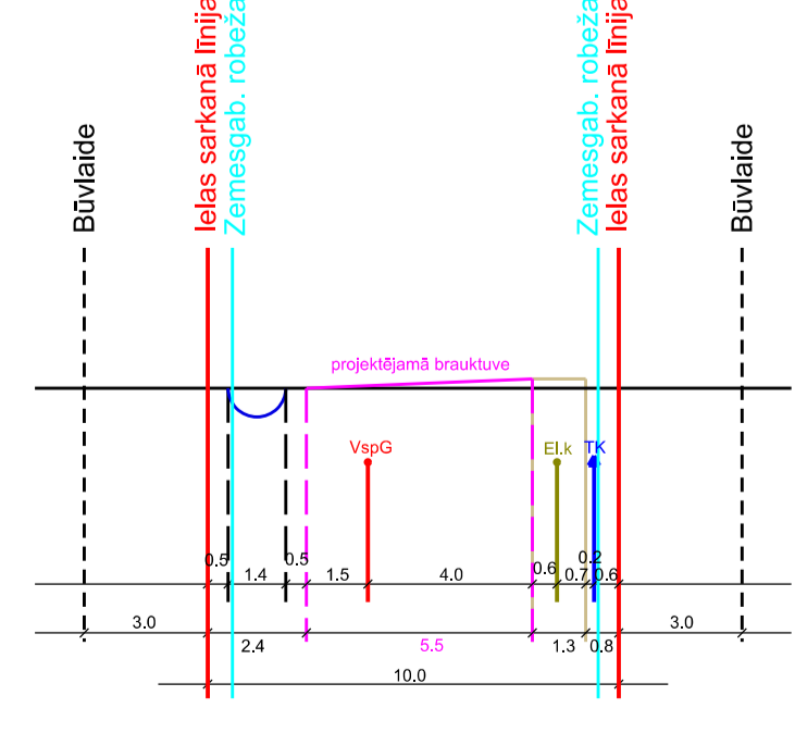
Seleriju ielas šķērsprofils 41-41 M 1:285
