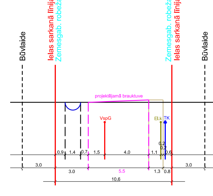
Seleriju ielas šķērsprofils 42-42 M 1:285
