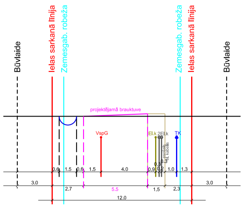
Līkloču ielas šķērsprofils 29-29 M 1:285
