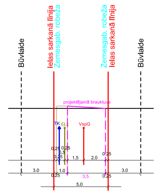
Mālu ielas šķērsprofils 35-35 M 1:285
