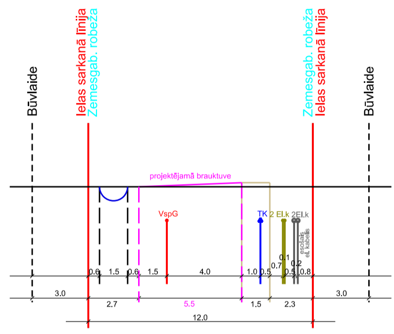
Līkloču ielas šķērsprofils 31-31 M 1:285
