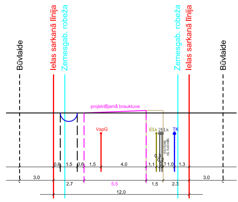
Līkloču ielas šķērsprofils 28-28 M 1:285
