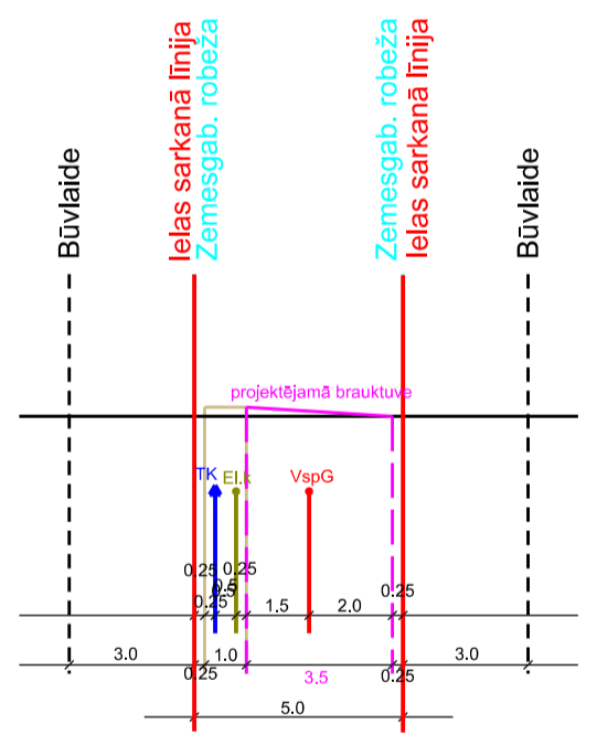
Mālu ielas šķērsprofils 36-36 M 1:285
