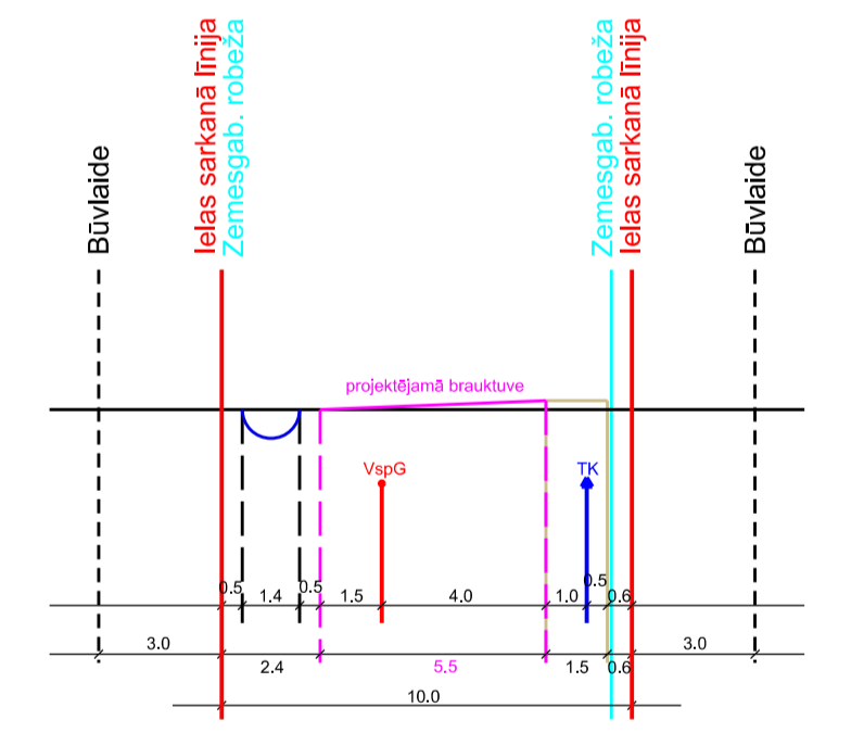
Līkloču ielas šķērsprofils 34-34 M 1:285
