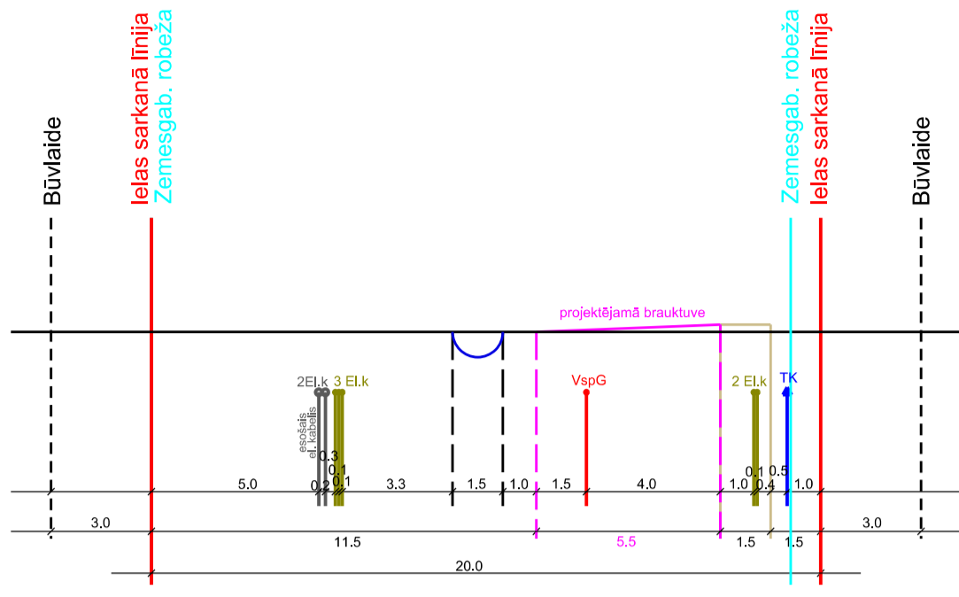
Bažciema ielas šķērsprofils 22-22 M 1:285
