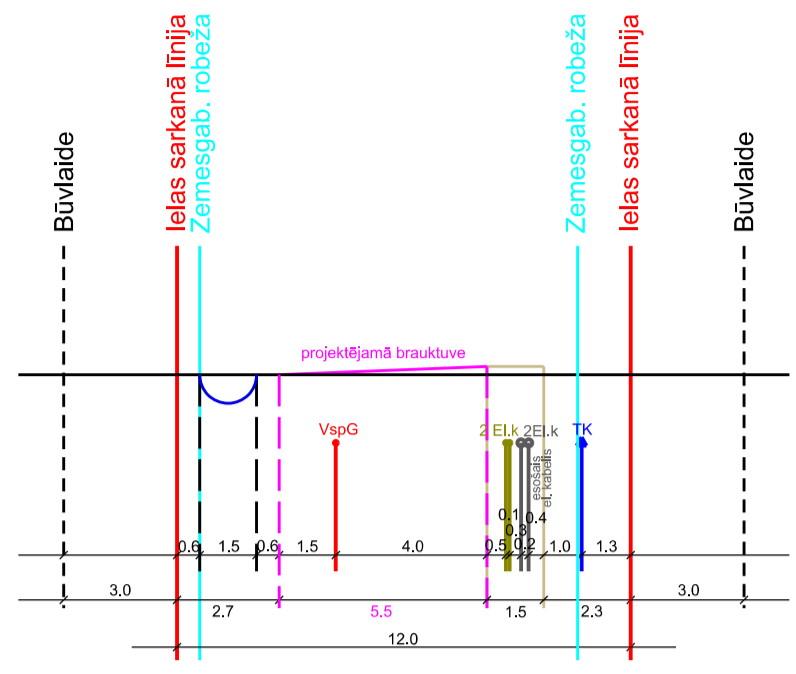
Līkloču ielas šķērsprofils 25-25 M 1:285
