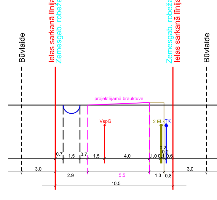
Seleriju ielas šķērsprofils 43-43 M 1:285
