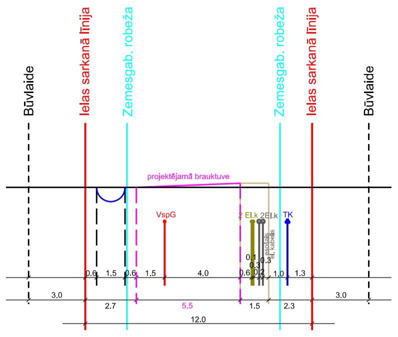
Līkloču ielas šķērsprofils 26-26 M 1:285
