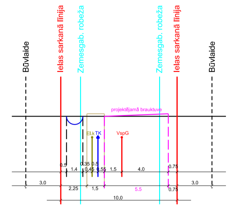
Līkloču ielas šķērsprofils 33-33 M 1:285
