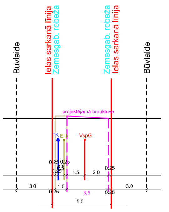
Pētersīļu ielas šķērsprofils 39-39 M 1:285
