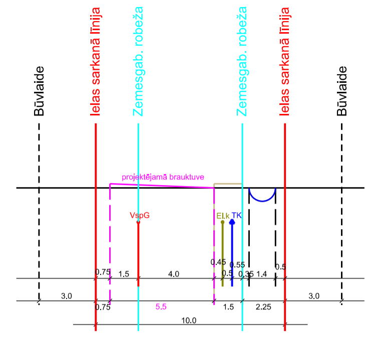
Maijpuķīšu ielas šķērsprofils 24-24 M 1:285
