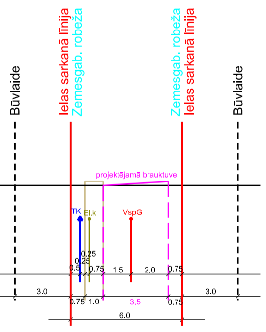
Mālu ielas šķērsprofils 37-37 M 1:285
