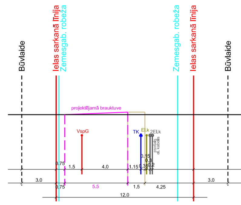
Līkloču ielas šķērsprofils 30-30 M 1:285
