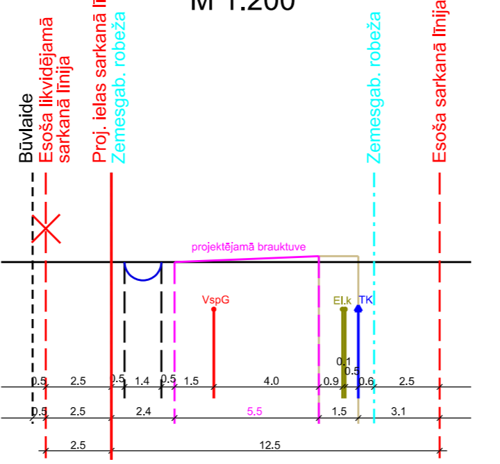
Sauļespuķu ielas šķērsprofils 64-64 M 1:200
