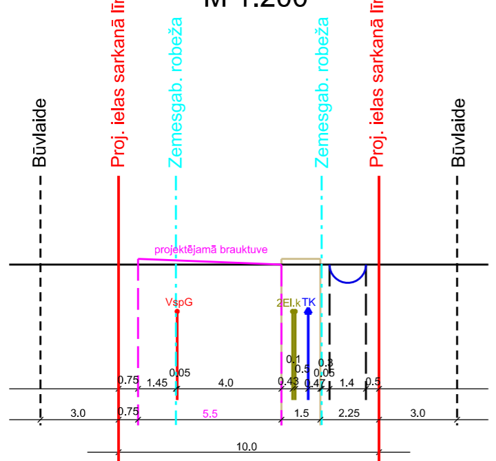
Līkloču ielas šķērsprofils 34-34 M 1:200
