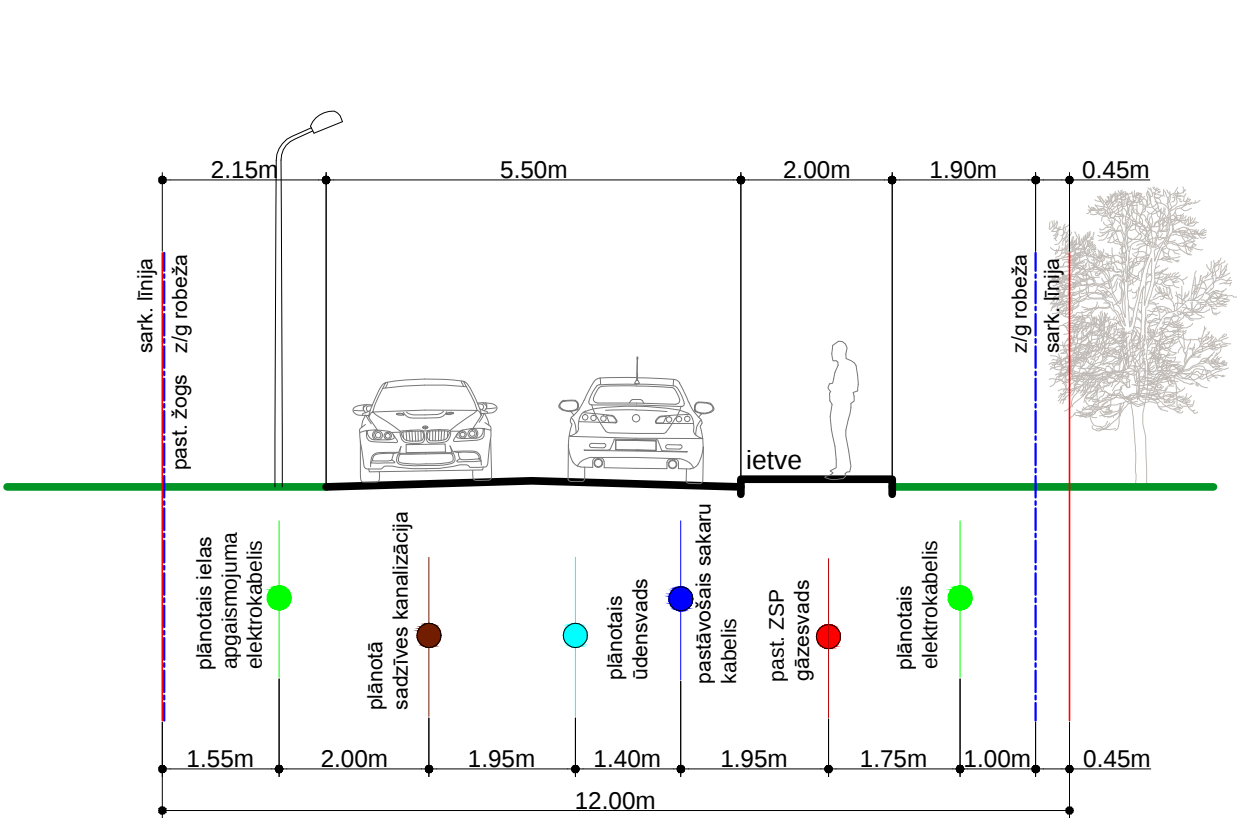
23. līnija, sarkanās līnijas 12,0m, E kategorijas iela, griezum B-B
