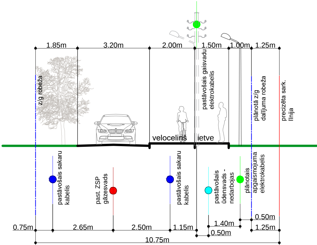
Rotas iela, sarkanās līnijas 12,0m, E kategorijas iela, griezum A-A
