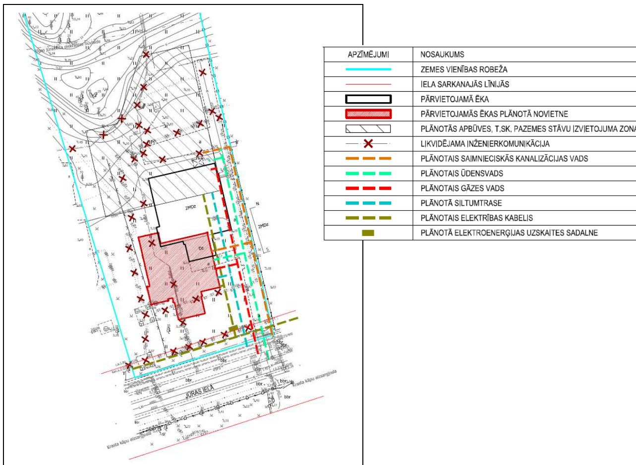
29.attēls. Plānotās inženierapgādes tīklu orientējošā izvietojuma shēma
