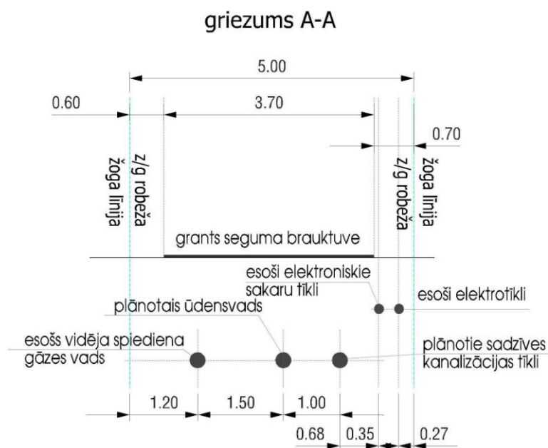
4.attēls. Satiksmes joslas šķēsgriezums ar esošām un plānotām inženierkomunikācijām.
