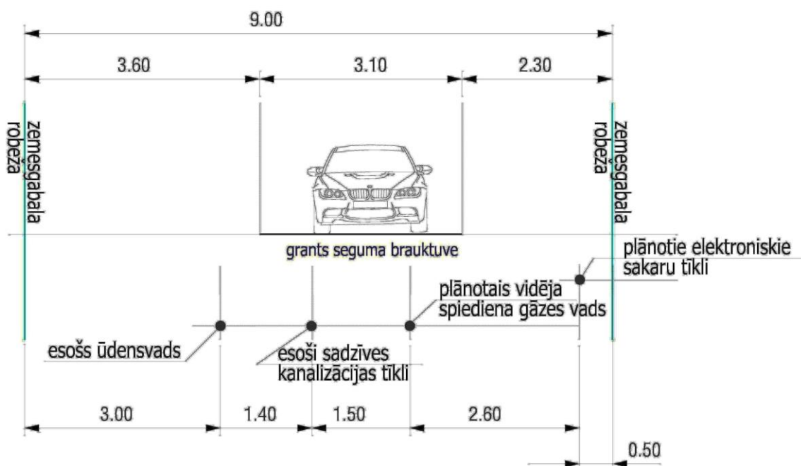
10. attēls. Satiksmes joslas šķērsprofils. Griezums A-A.
