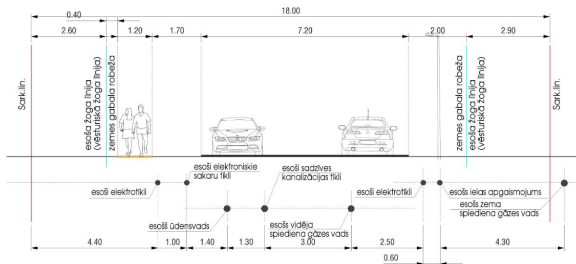
13.attēls. Esošs Kāpu ielas šķēršprofils.. Griezums A-A.
