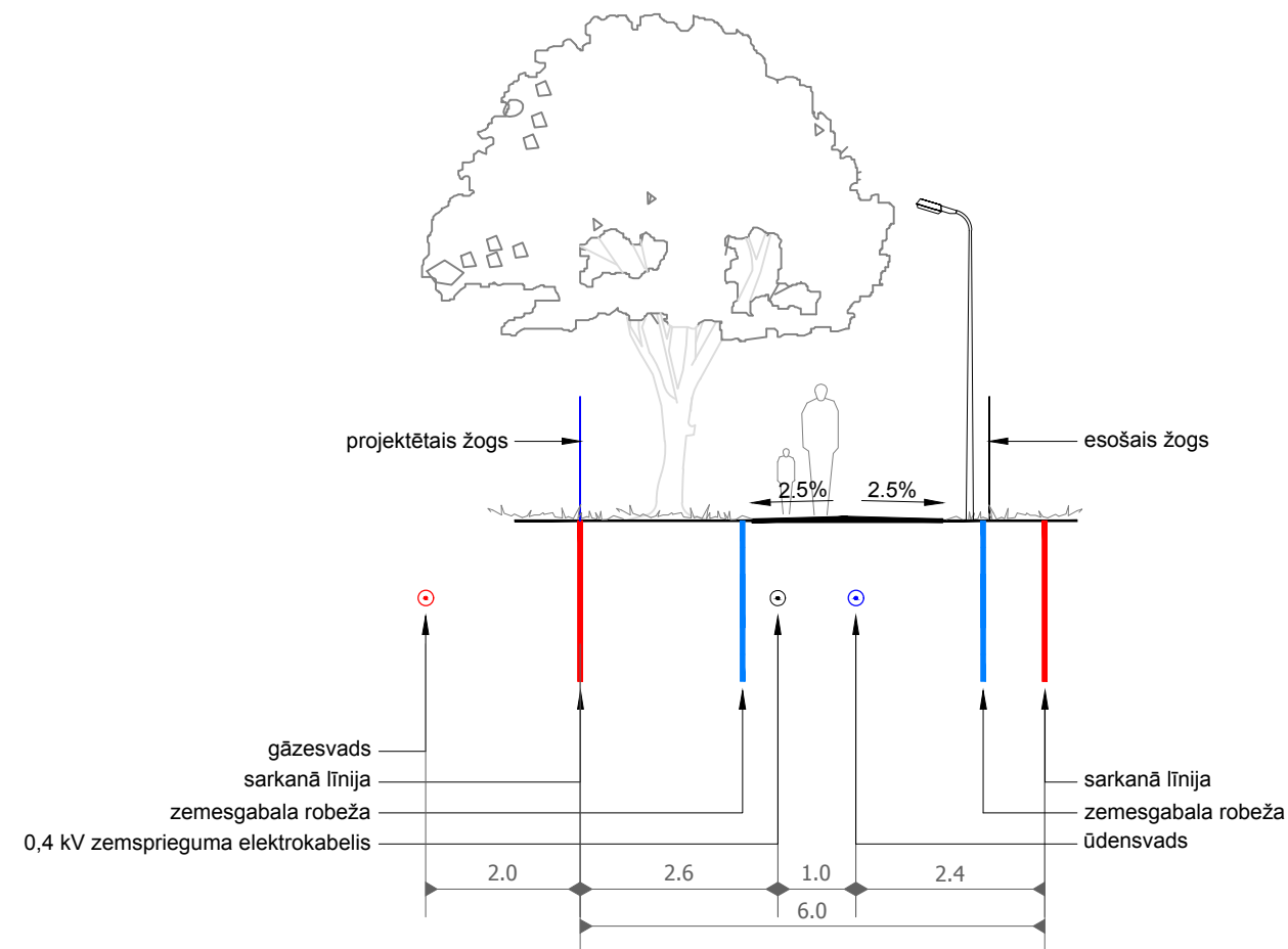
ASPAZIJAS IELA 2, SARKANĀS LĪNIJAS 6.0m 'E' KATEGORIJAS IELA GRIEZUMS A-A M 1:100 PROJEKTĒTAIS
