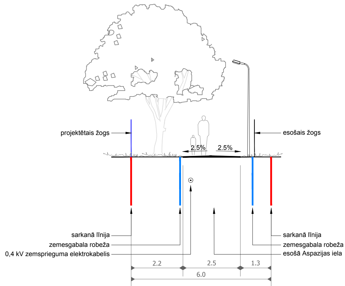
ASPAZIJAS IELA 2, SARKANĀS LĪNIJAS 6.0m 'E' KATEGORIJAS IELA GRIEZUMS A-A M 1:100 ESOŠAIS
