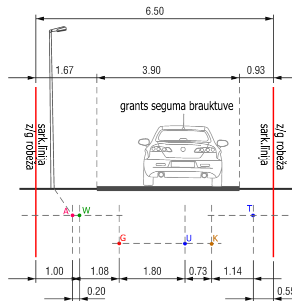
KRŪMU ielas sarkanās līnijas 6.5m griezumums B - B (esošs)
