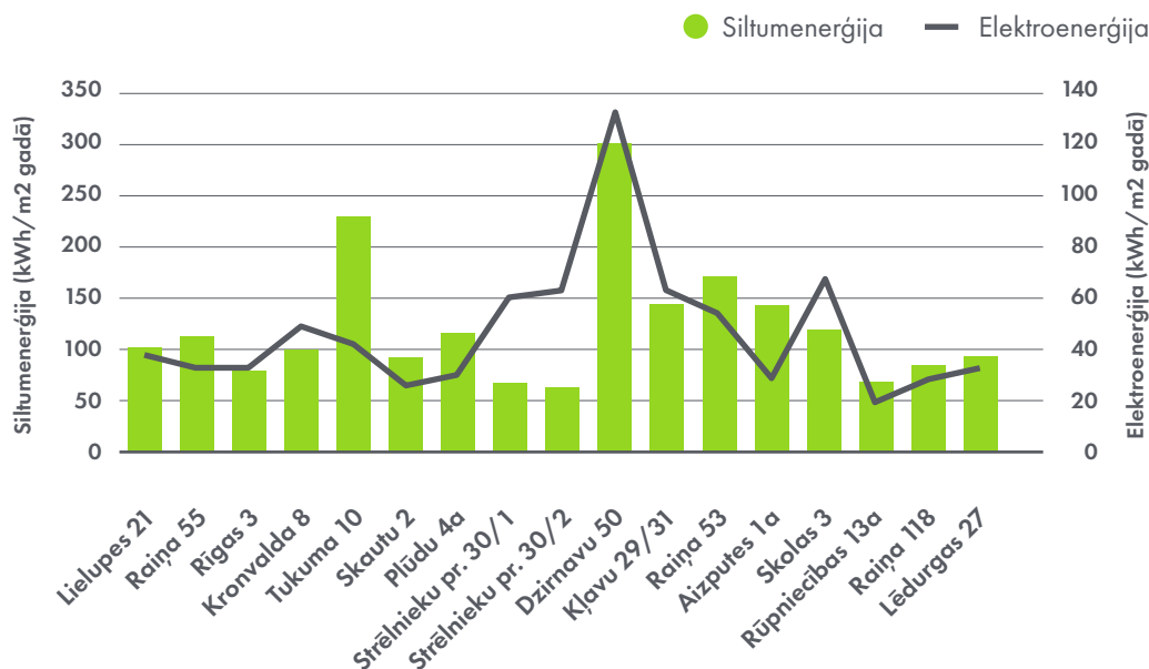
9. attēls. Enerģijas patēriņš skolās (vidēji 2018.–2020. gadā)
