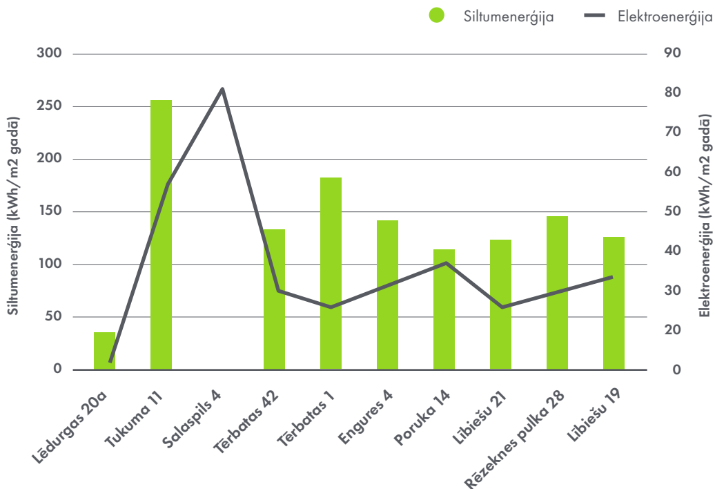
8. attēls. Enerģijas patēriņš pirmsskolas izglītības iestādēs (vidēji 2018.–2020. gadā)
