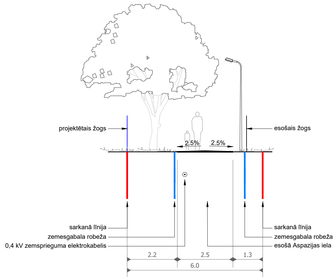
ASPАЗIJAS IELA 2, SARKANĀS LĪNIJAS 6.0m 'E' KATEGORIJAS IELA GRIEZUMS A-A M 1:100 ESOŠAIS
