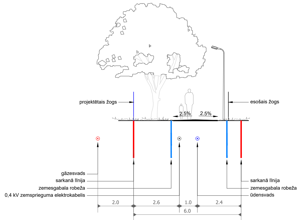
ASPАЗIJAS IELA 2, SARKANĀS LĪNIJAS 6.0m 'E' KATEGORIJAS IELA GRIEZUMS A-A M 1:100 PROJEKTĒTAIS
