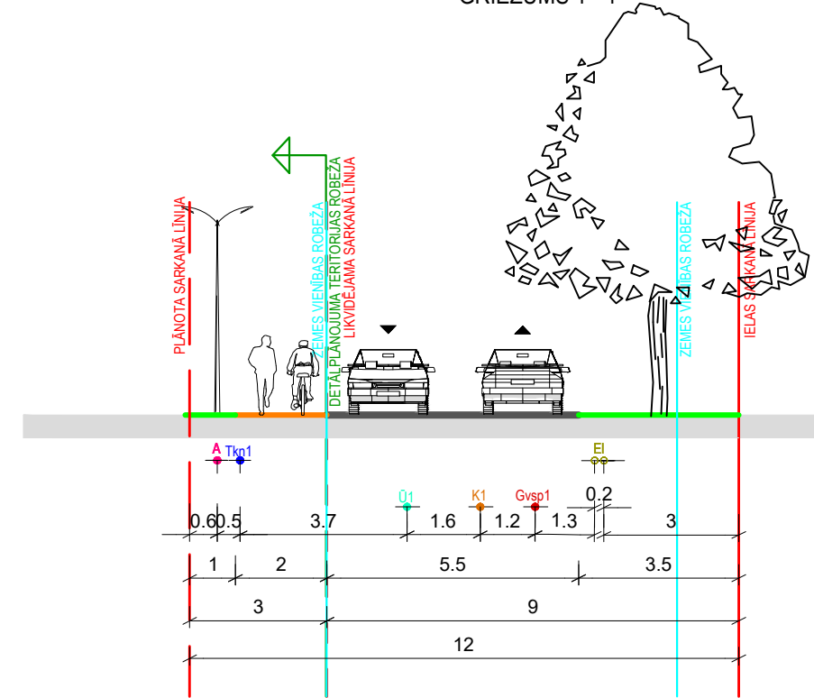
TEĀTRA IELAS POSMA A ŠĶĒRSPROFILS GRIEZUMS 1 - 1
