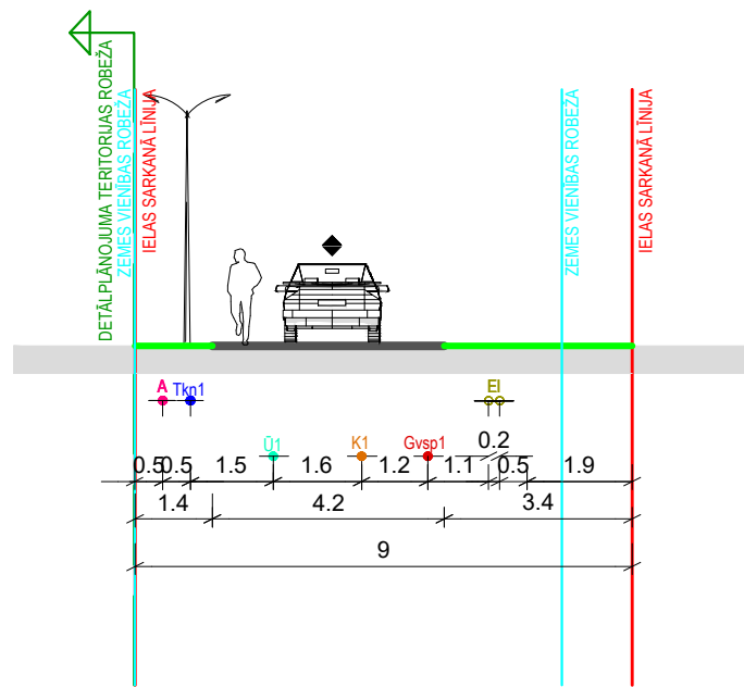
TEĀTRA IELAS POSMA B ŠĶĒRSPROFILS GRIEZUMS 2 - 2
