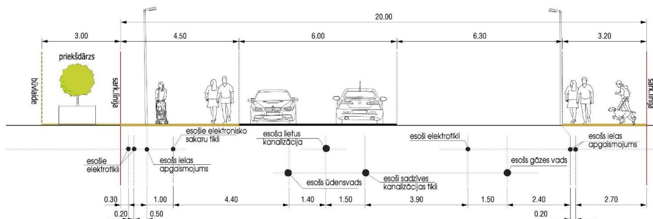
46.attēls. Turaidas ielas šķērsgriezums. Griezums A-A. Sarkano līniju platums 20 metri.
